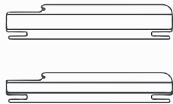
KASA ENKESİT GÖRÜNÜMLERİ / JAMB CROSS - SECTION VIEW
